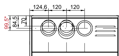
Vista frontale
