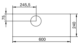
Vista dall'alto
