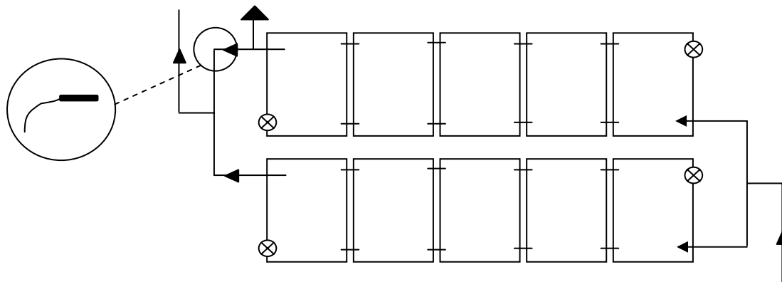
Пример за паралелно свързване в редове
